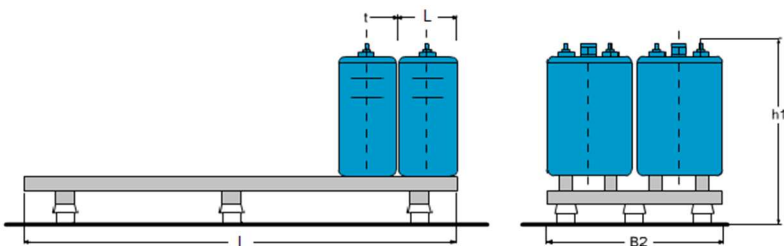
Двухрядные стеллажи
