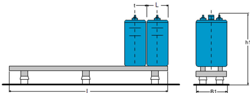
Однорядные стеллажи
