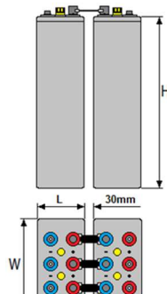
OGi1520 ÷ OGi2400
