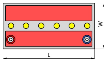
6 x 1 OPzS 50 6 x 2 OPzS 100 6 x 3 OPzS 150
